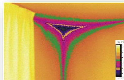
Pierderea căldurii la colțul încăperii
